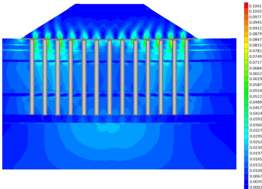
Рис. 3. Распределение относительных деформаций в грунтовом массиве при устройстве насыпи на укрепленном основании.
